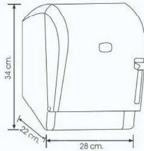
Autocut Roll Paper Towel Dispenser Autocut Rulo Kağıt Havlu Dispenseri
