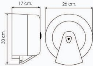
centerpoint Toilet Tissue Dispenser İçten Çekmeli Tuvalet Kağıdı Dispenserli
